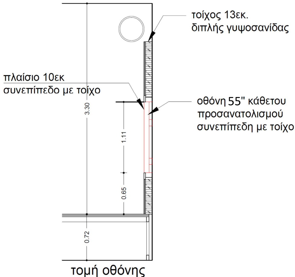
Εικόνα 20: Ενδεικτική τομή εγκατεστημένης διαδραστικής οθόνης αφής (B7).
