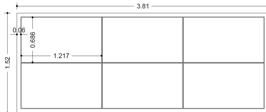
Εικόνα 14: Κάτοψη μεγάλου διαδραστικού τραπέζιού.
