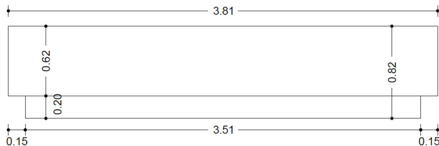
Εικόνα 15: Όψη μεγάλου διαδραστικού τραπέζιού.
