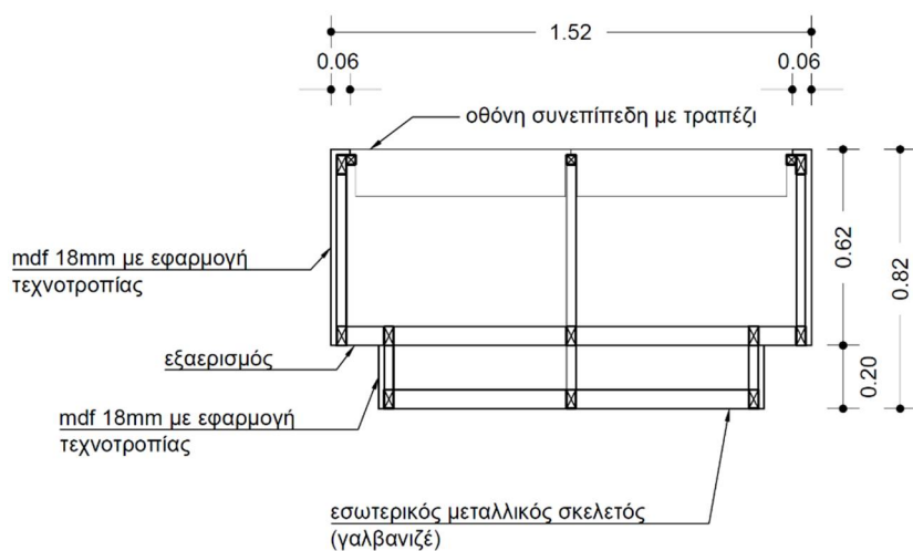
Εικόνα 16: Όψη μεγάλου διαδραστικού τραπέζιού.
