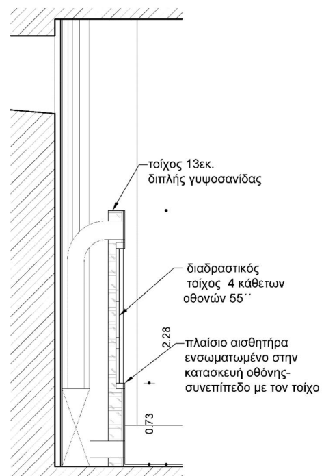
τομή διαδραστικού τοίχου
