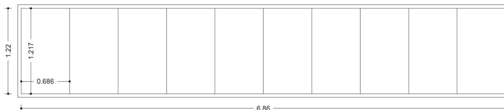
Εικόνα 10: Ενδεικτικό σχέδιο του διαδραστικού τοίχου B 1 .
