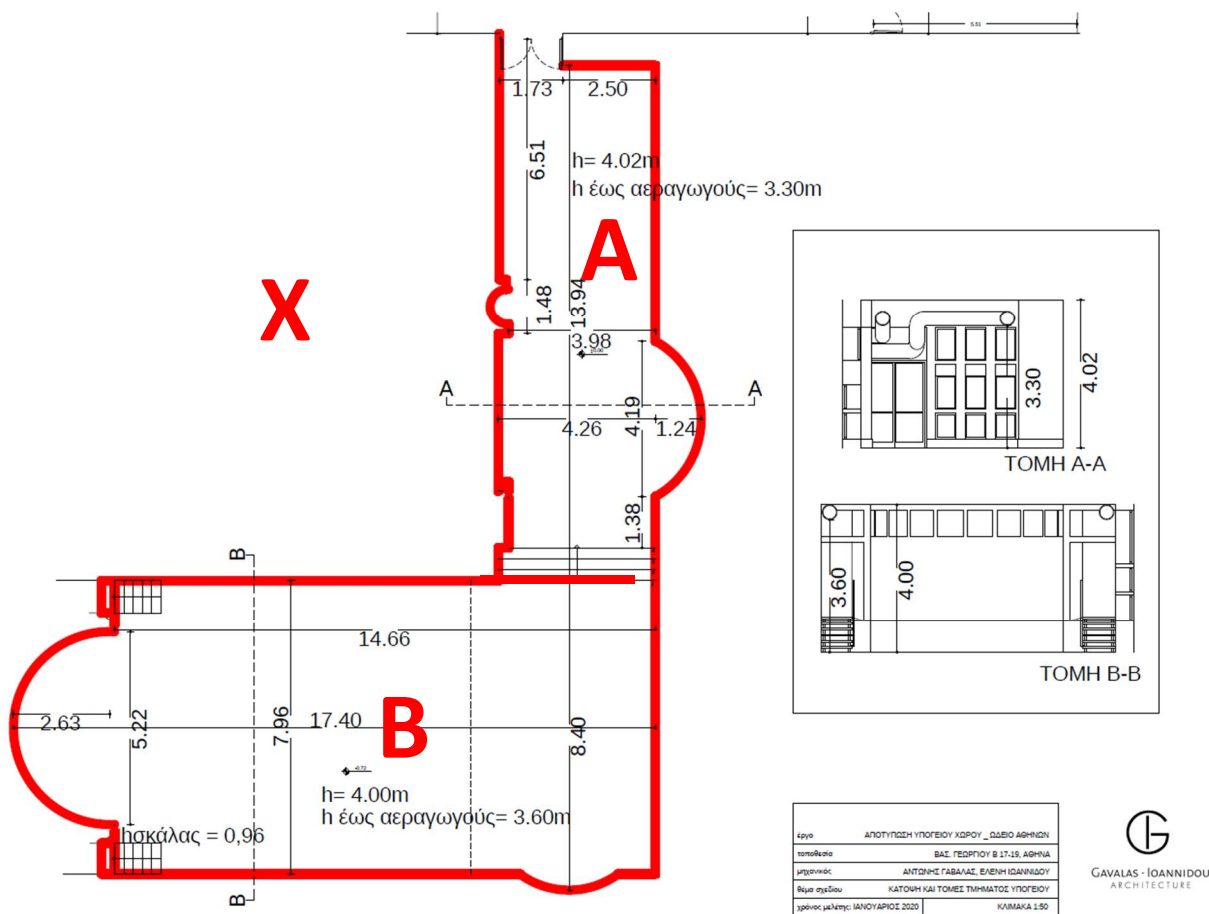
Εικόνα 1: Κάτοψη του χώρου που θα μετατραπεί σε ψηφιακό/βιωματικό, στο επίπεδο -1 του Ωδείου Αθηνών.
