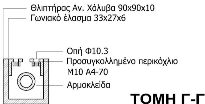
Εικ. 5 Λεπτομέρεια διαμόρφωσης θλιπτήρα (τομές Α-Α, Β-Β, Γ-Γ και κάτοψη)
