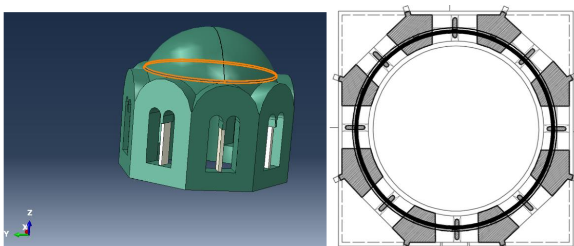
Εικ. 7 Ενδεικτική διάταξη της θέσης της αφανούς μεταλλικής περίδεσης του ναού
