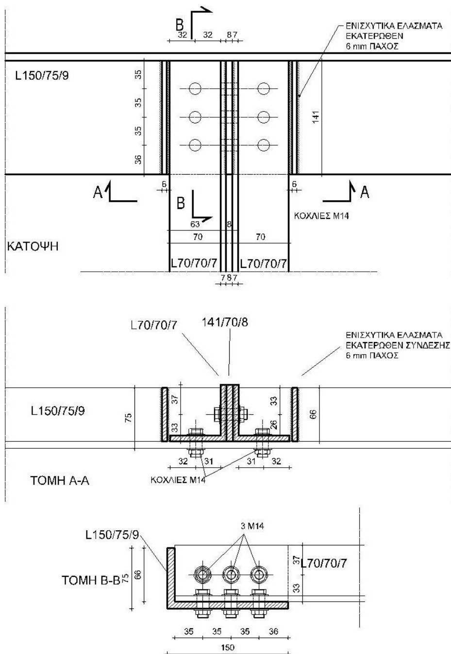
Εικ. 12 Λεπτομέρεια διαμόρφωσης των κοχλιωτών συνδέσεων μεταξύ των μελών των καμπύλων διαφραγματικών διατάξεων (σύνδεση στρωτήρα με κύρια δοκό)
