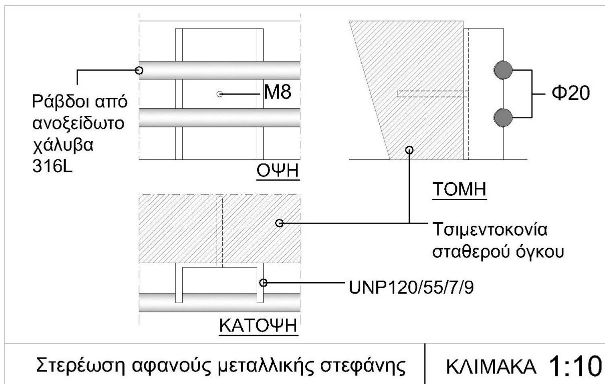
Εικ. 8 Λεπτομέρεια διαμόρφωσης της αφανούς μεταλλικής περίδεσης του τρούλου του ναού
