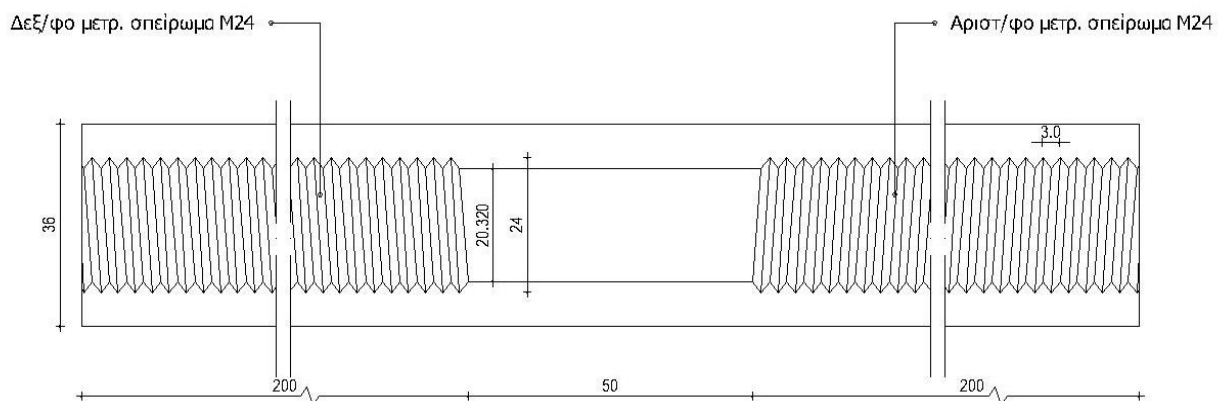
Εικ.3 Λεπτομέρειες διαμόρφωσης σπειρωμάτων και αρμοκλείδας τάνυσης ελκυστήρων Φ25
