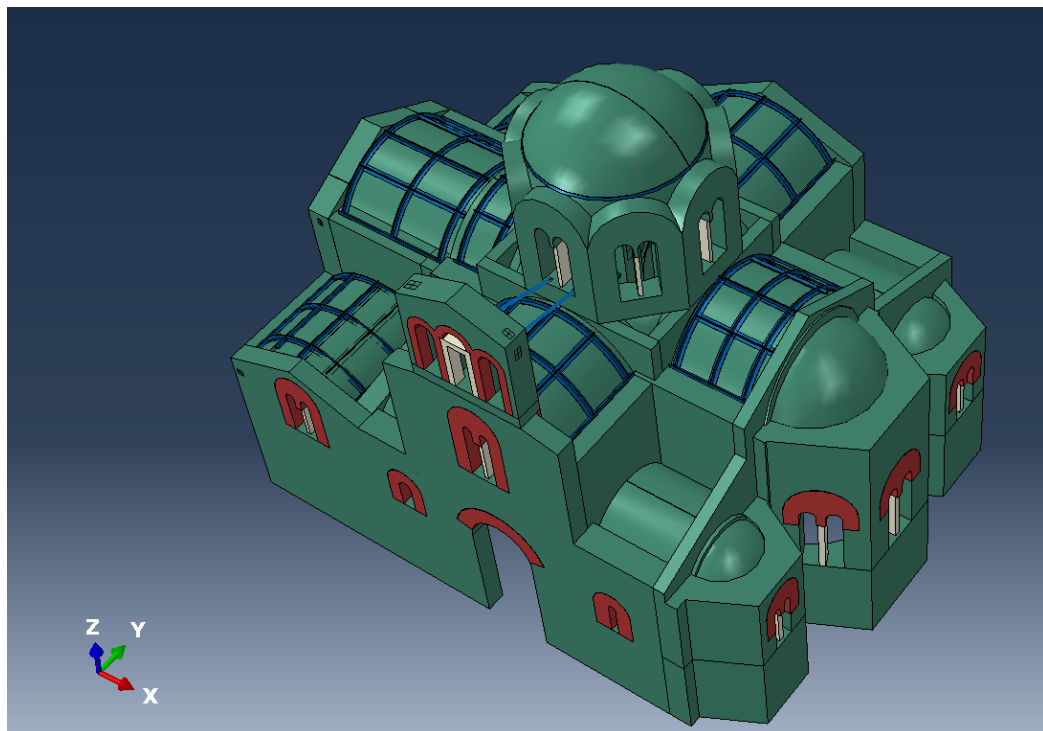
Εικ. 10 Ενδεικτική απεικόνιση της διάταξης των θολωτών μεταλλικών ενισχύσεων στα εξωράχια των θόλων
