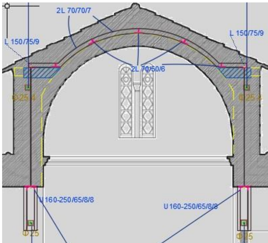
Εικ. 11 Ενδεικτική απεικόνιση και κατακόρυφη τομή της διάταξης των θολωτών μεταλλικών ενισχύσεων
