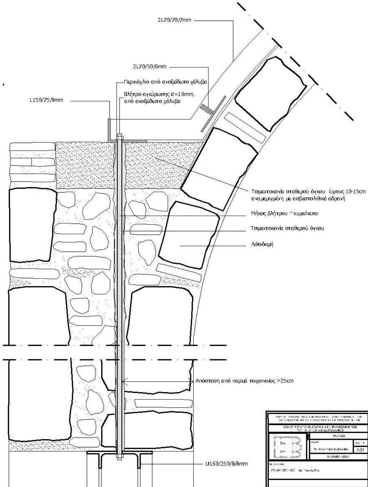
Εικ. 15 Λεπτομέρεια διαμόρφωσης της σύνδεσης μεταξύ θολωτών διαφραγματικών διατάξεων εξωραχίων και ανοξείδωτων μεταλλικών καμπύλων διατομών περίσφιξης των κατακόρυφων εδράσεων των θόλων
