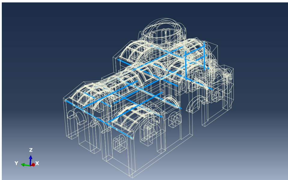
Εικ. 1 Θέσεις προτεινόμενων νέων ελκυστήρων και αγκυρίων εντός του ναού
