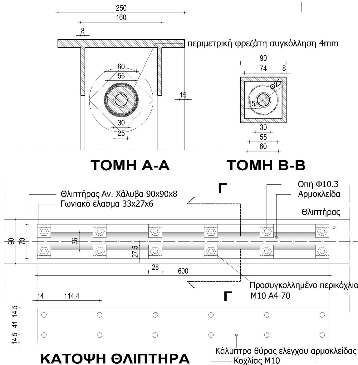
Εικ. 4 Λεπτομέρεια σύνδεσης θλιπτήρα με τα σημεία στήριξής του επί των καμπύλων διατομών περισφίξης
