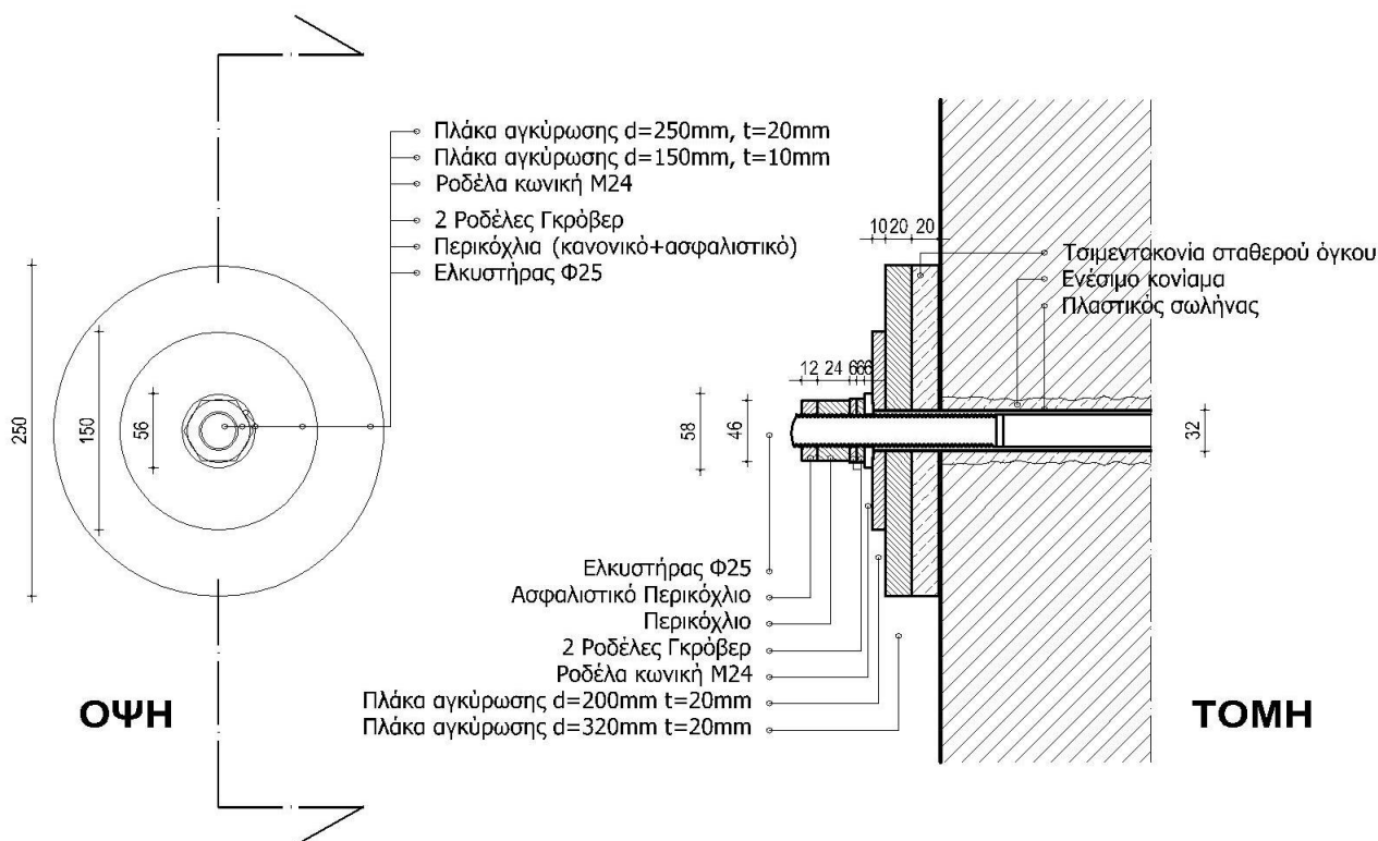
Εικ. 6 Λεπτομέρεια διαμόρφωσης της αγκύρωσης των ελκυστήρων Φ25 στους εξωτερικούς τοίχους του ναού
