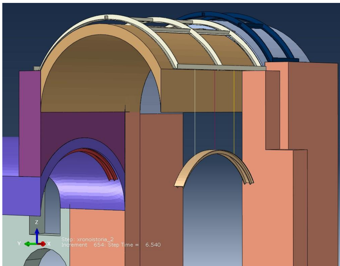
Εικ. 14 Ενδεικτική απεικόνιση της διάταξης των καμπύλων ενισχυτικών διατομών περίσφιξης και η σύνδεσή τους με τις θολωτές μεταλλικές ενισχύσεις στο προσομοίωμα του φορέα του ναού
