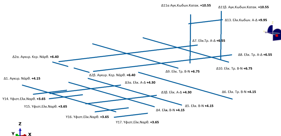
Εικ. 2 Κωδικοποίηση και στάθμες υφιστάμενων και νέων ελκυστήρων-αγκυρίων
