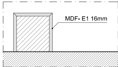
Ενδεικτική τομή B2 1:10
