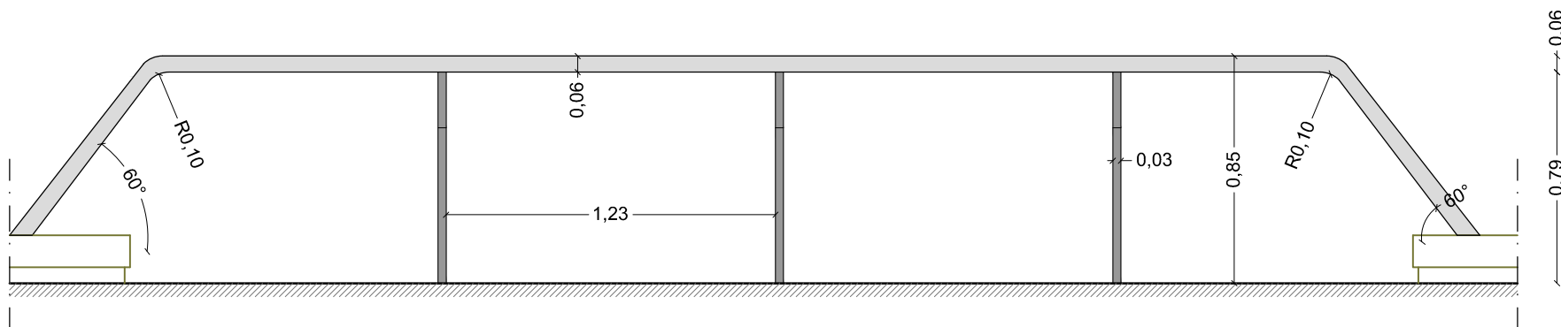
Πρόσοψη 1:25
