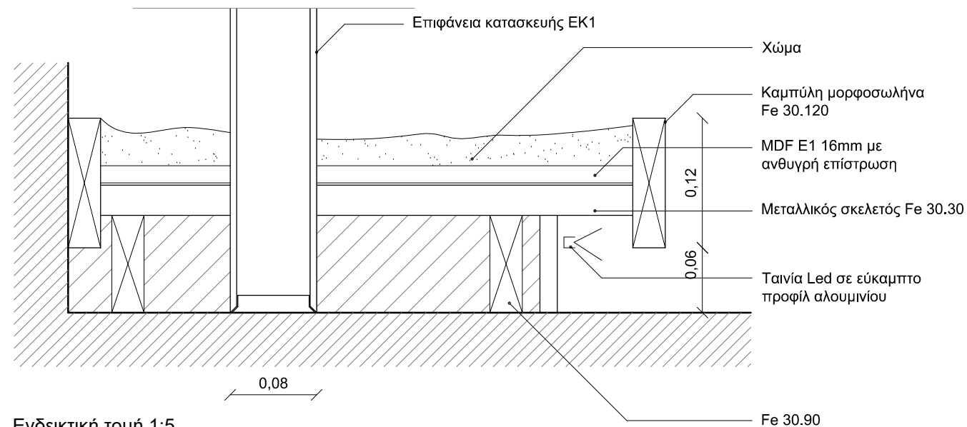
Ενδεικτική τομή 1:5
