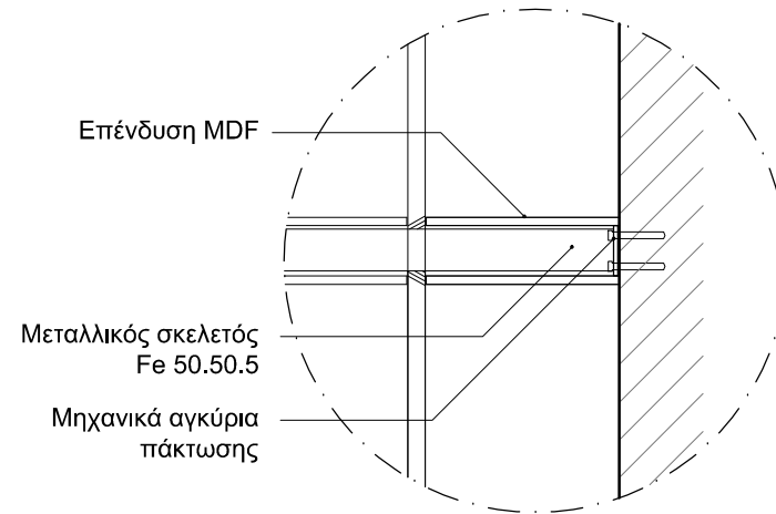
Λεπτομέρεια 2 1:10
