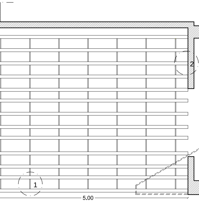
Κάτοψη 1:50
