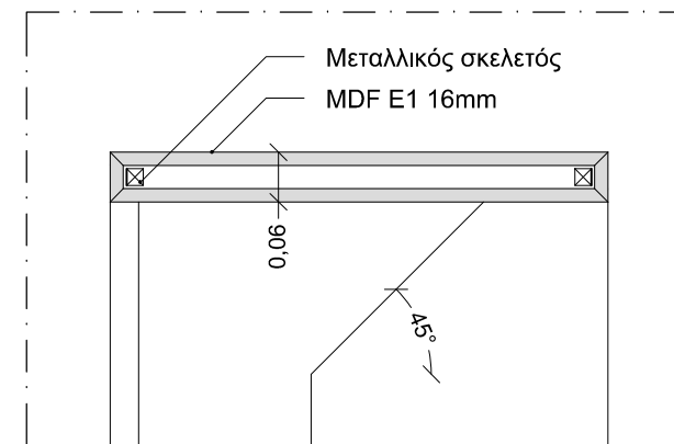
Λεπτομέρεια τομής 1:10
