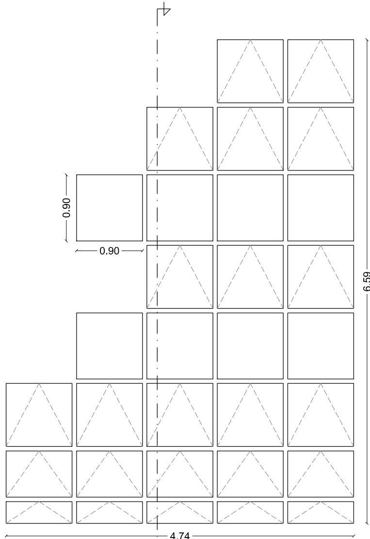
Κάτοψη συνολικής κατασκευής 1:50
