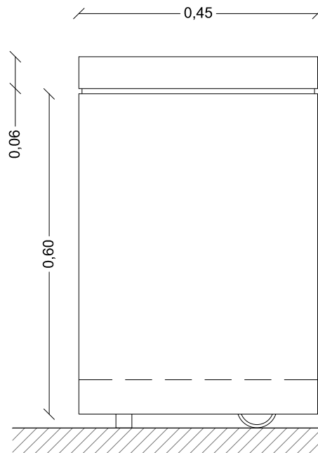
Πλάγια όψη
