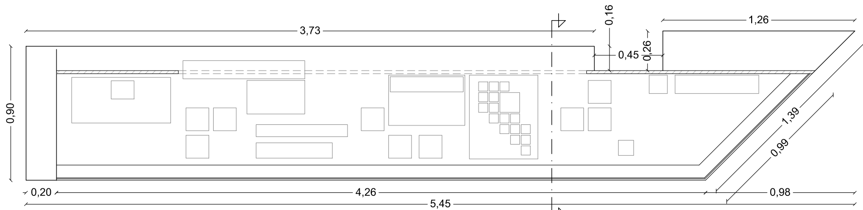
Κάτοψη 1:25
