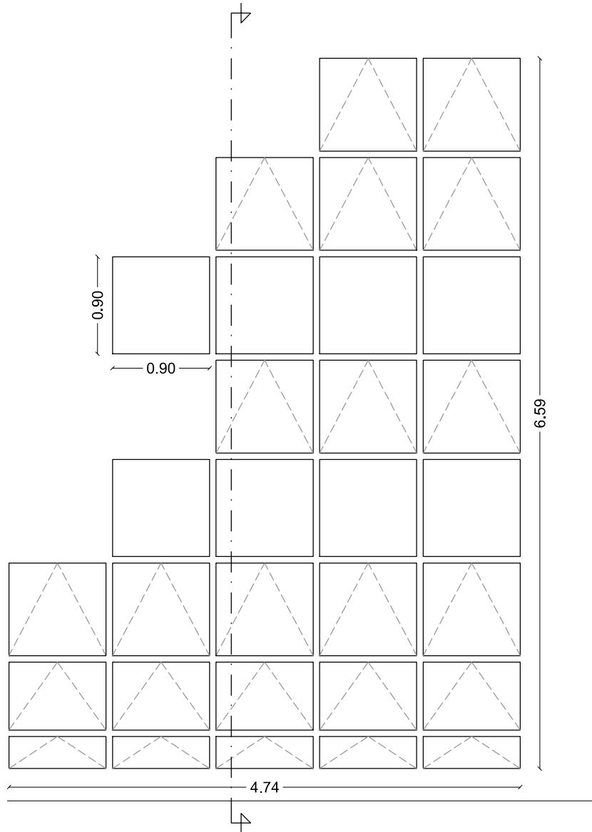
Κάτοψη συνολικής κατασκευής 1:50
