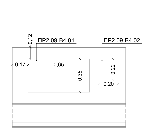
Κάτοψη
