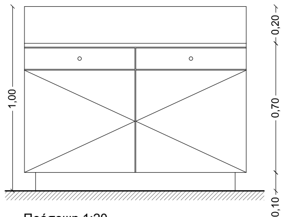
Πρόσοψη 1:20
