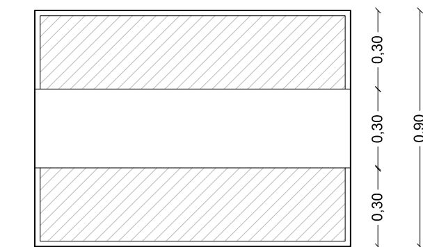
Κάτοψη 1:20
