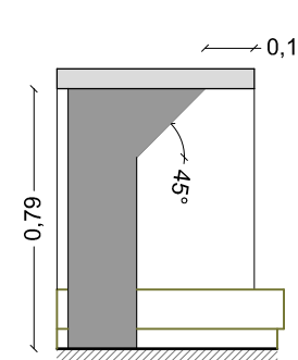
Τομή 1:25
