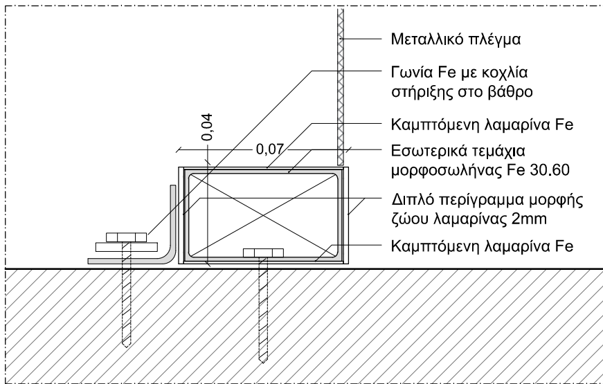
Λεπτομέρεια 1:2
