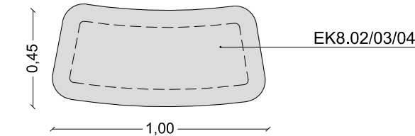
Κάτοψη 1:25
