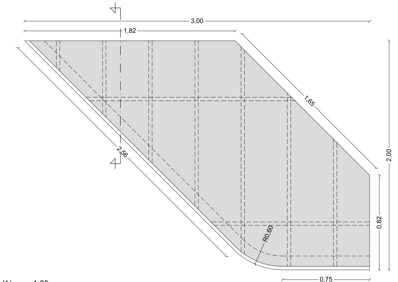
Κάτοψη 1:20
