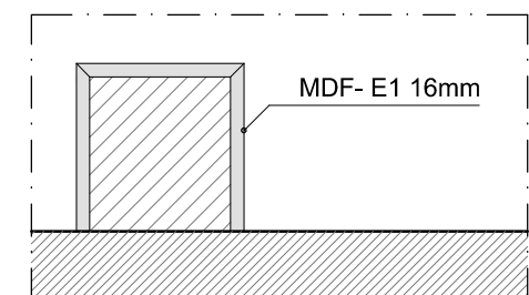
Ενδεικτική τομή B2 1:10
