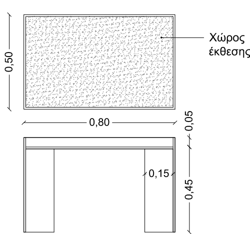
Ενδεικτική λεπτομέρεια Β3
