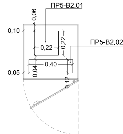
Κάτοψη
