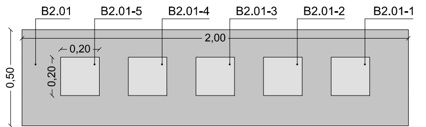
Κάτοψη 1:20
