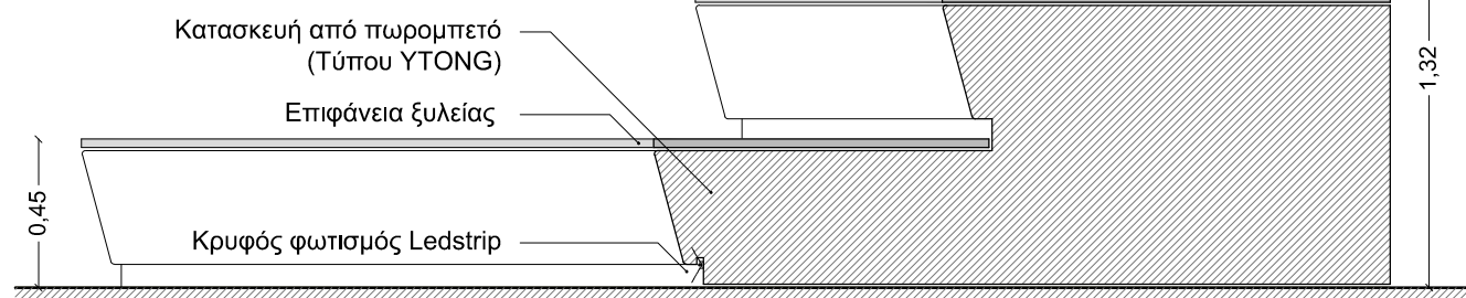
Τομή 1:25
