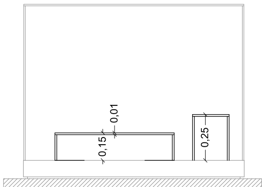
Πρόσοψη
