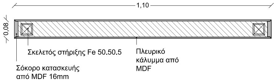
Τομή Α-Α' 1:10
