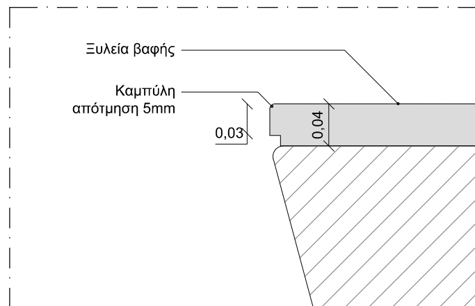
Λεπτομέρεια 1:5
