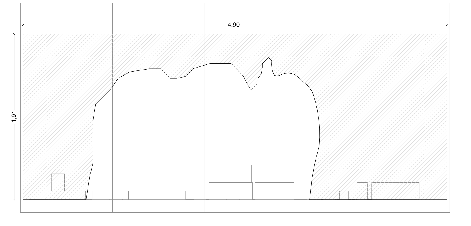
Πρόσοψη 1:25
