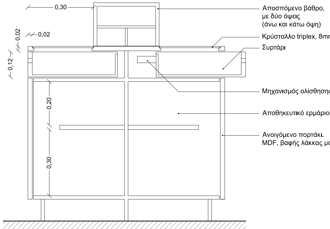
Τομή 1:10
