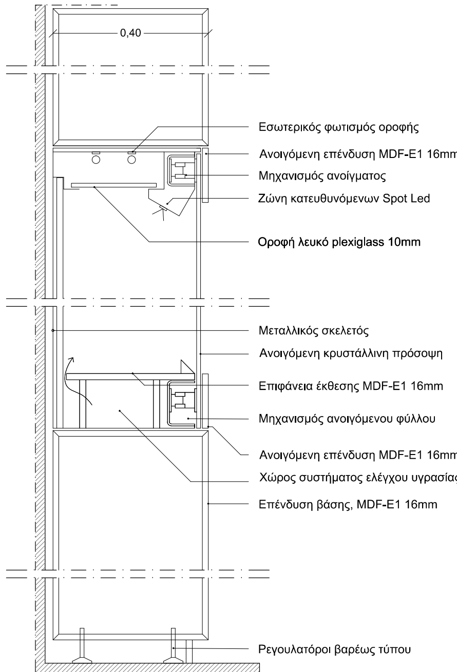
Τομή 1:10
