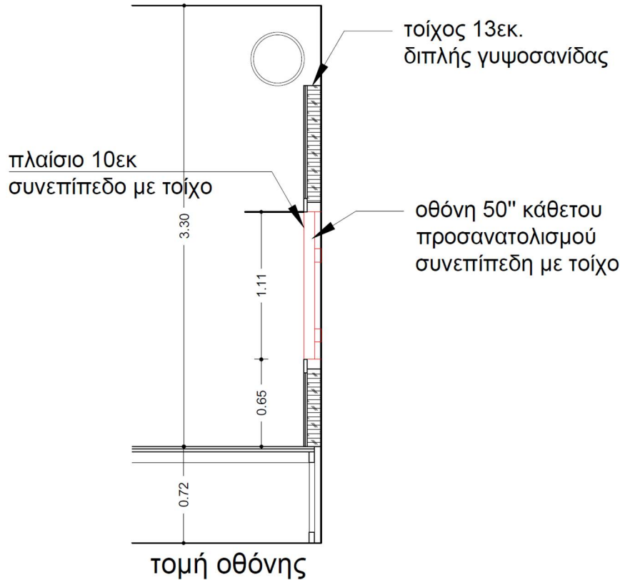
Εικόνα 15: Ενδεικτική τομή εγκιβωτισμένης διαδραστικής οθόνης αφής ( B_7 ). Οι τελικές διαστάσεις μπορεί να κυμαίνονται μεταξύ 1,2 και 1,5 μέτρα ύψος.
