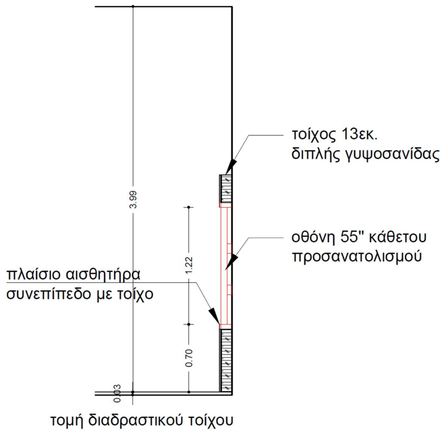
Εικόνα 11: Ενδεικτική τομή του διαδραστικού τοίχου B 1 (εγκιβωτισμένου σε τοίχο από γυψοσανίδα). Οι τελικές διαστάσεις μπορεί να κυμαίνονται μεταξύ 1,2 και 1,5 μέτρα ύψος.
