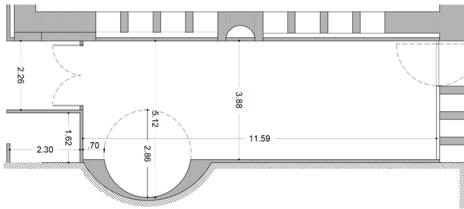
Εικόνα 4: Κάτοψη του χώρου των κινήτρων. Το ύψος του χώρου είναι τέσσερα (4) μέτρα.
