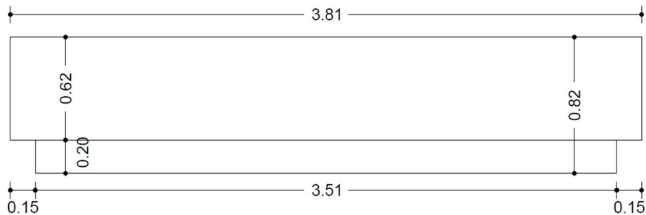
Εικόνα 13: Όψη μεγάλου διαδραστικού τραπέζιού.
