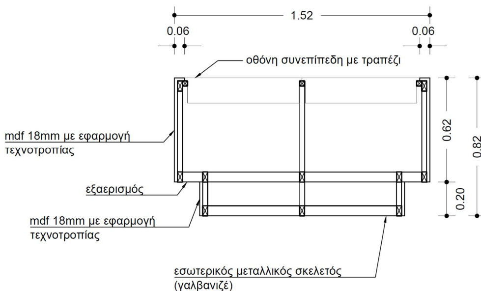
Εικόνα 14: Όψη μεγάλου διαδραστικού τραπέζιού.
