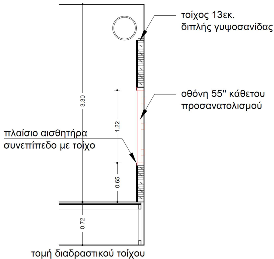
Εικόνα 9: Ενδεικτική τομή του διαδραστικού τοίχου B_1 (εγκιβωτισμένου σε τοίχο από γυψοσανίδα). Οι τελικές διαστάσεις μπορεί να κυμαίνονται μεταξύ 1,2 και 1,5 μέτρα ύψος.
