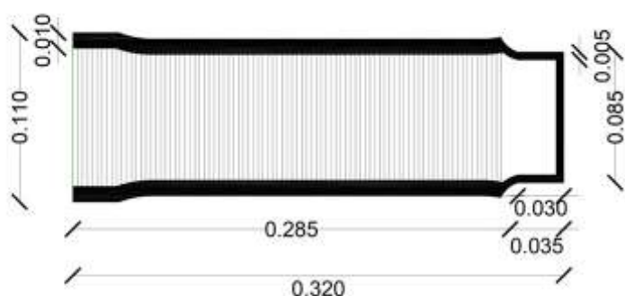
ΤΟΜΗ ΠΗΛΟΣΩΛΗΝΑ (ΔΙΑΣΤΑΣΕΙΣ ΣΕ ΜΕΤΡΑ)
