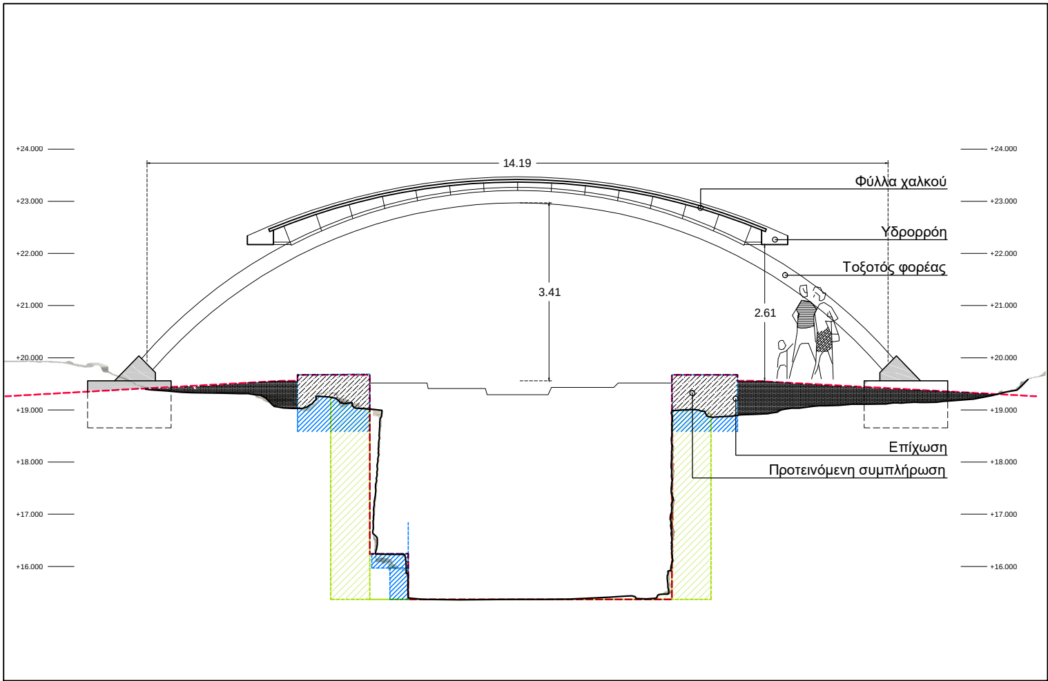
ΤΟΜΗ Ε2
