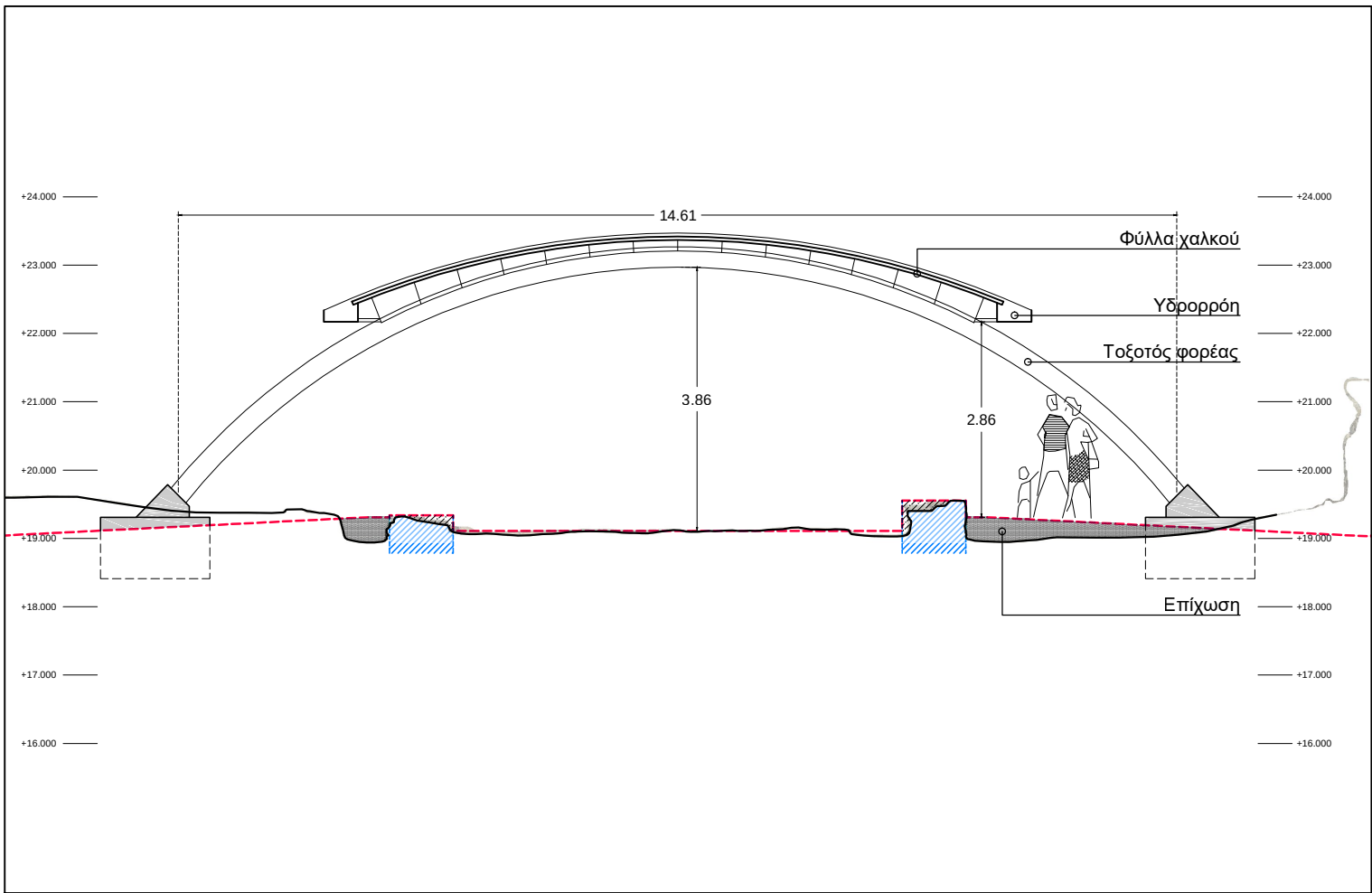
ΤΟΜΗ Ε1
